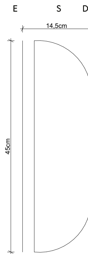
ARANDELA DONUT 1:5
