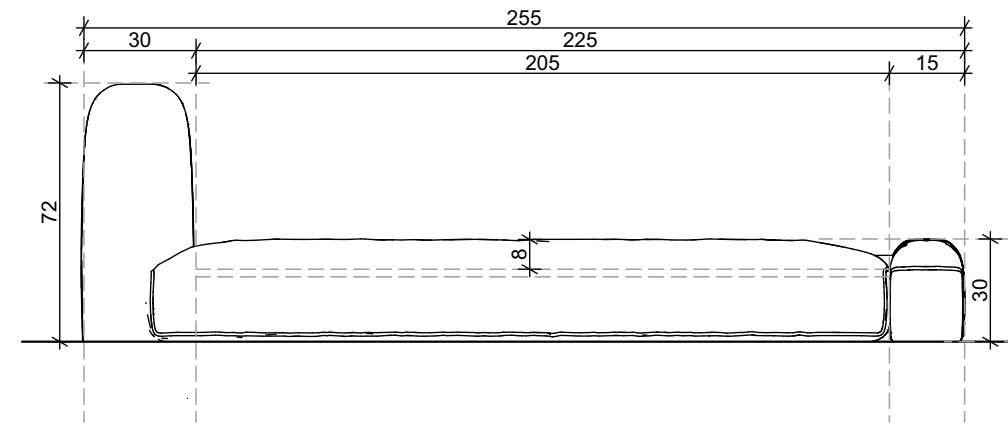
CAMA GÁRGULA 1:20
