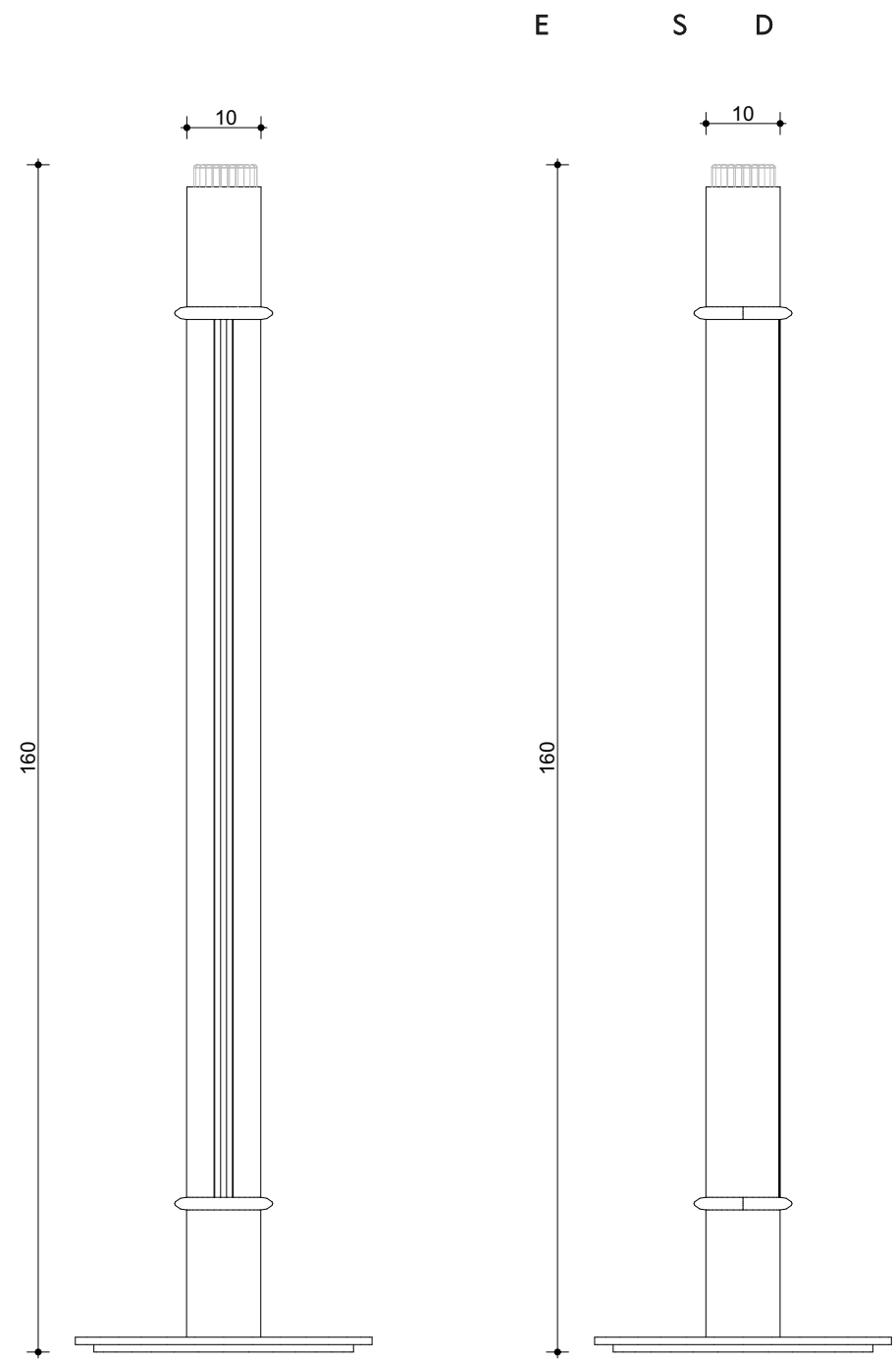
COLUNA DUCTO 1:10
