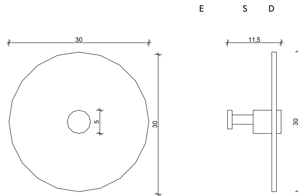
LUMINÁRIA BOTÃO CIRCULAR 1:5
