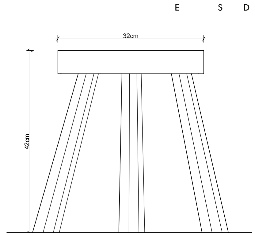
BANCO ORDENHA RETANGULAR 1:5
