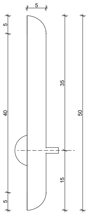
LUMINÁRIA CANOA 1:5
