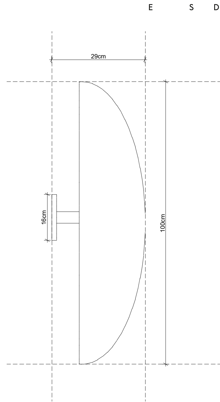
LUMINÁRIA ESPELHO (G) 1:5
