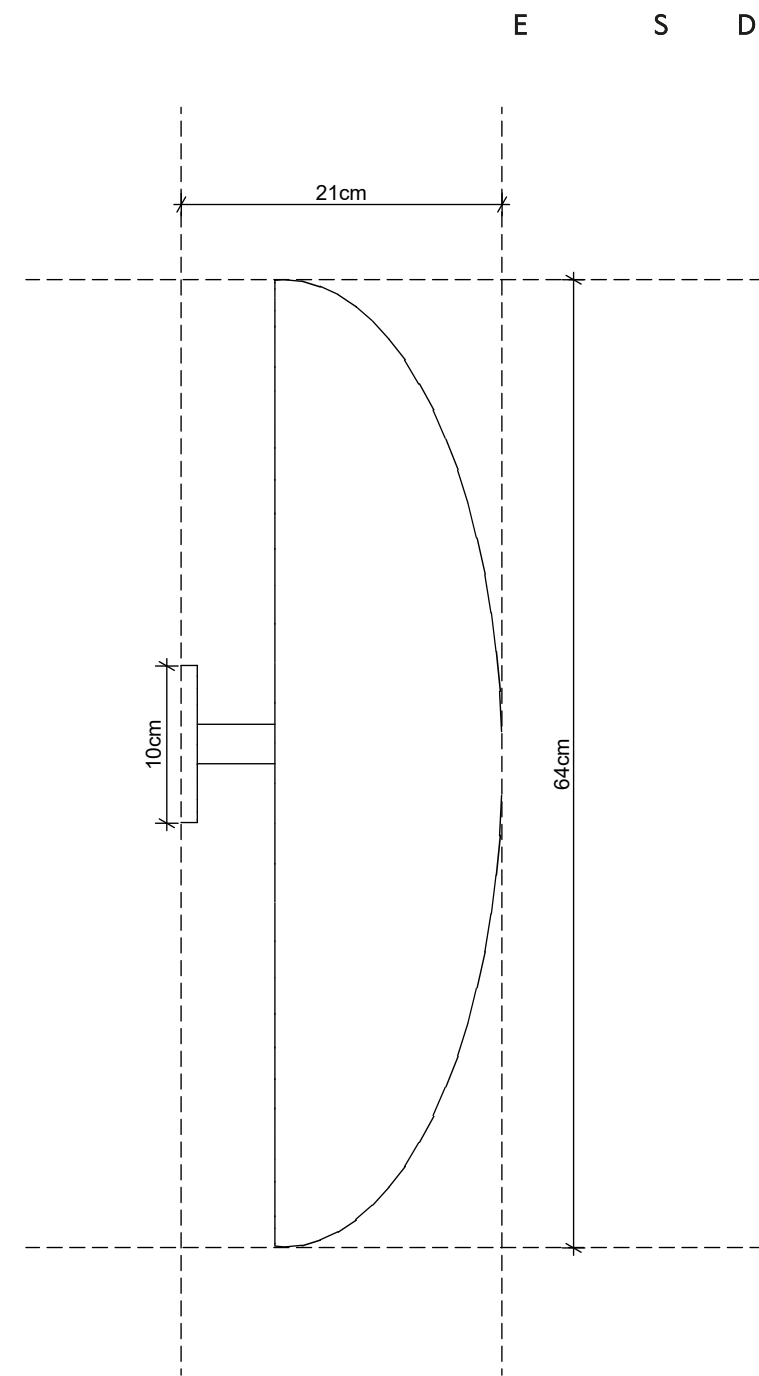
LUMINÁRIA ESPELHO (P) 1:5
