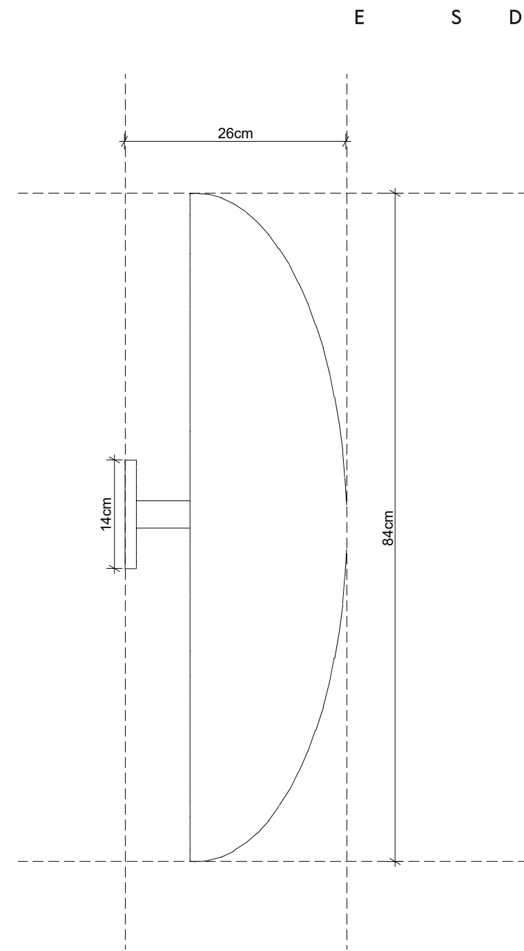
LUMINÁRIA ESPELHO (M) 1:5
