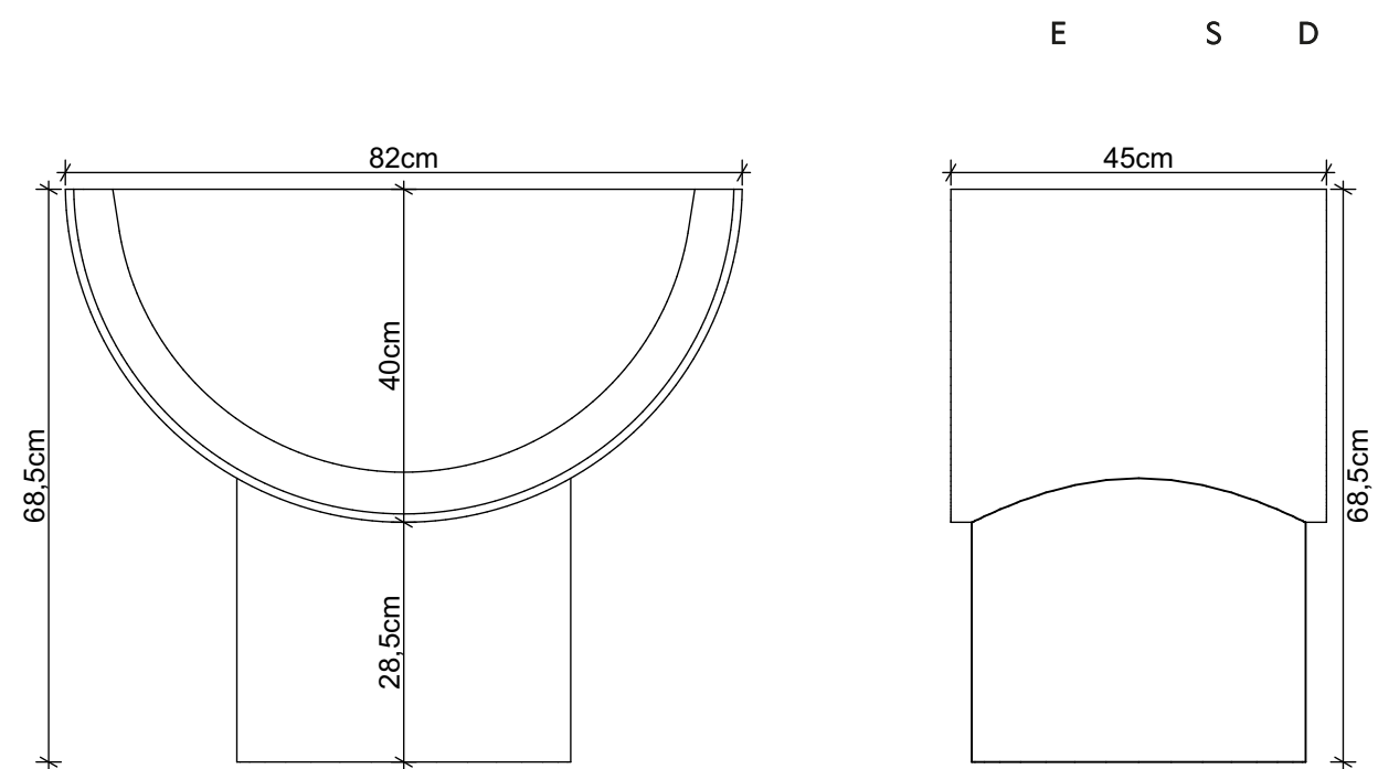
POLTRONA CÔNCAVO 1:1
