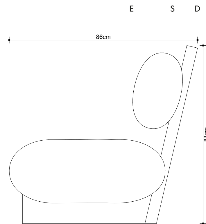
POLTRONA SALA 1:10
